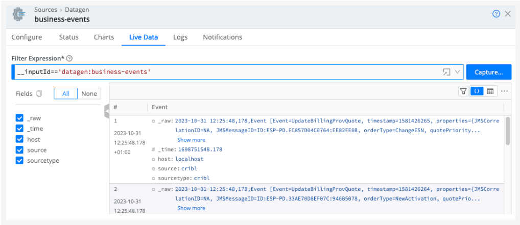
Source modal > Live Data tab
